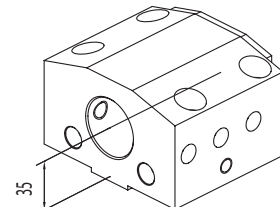
PU1-32-40 Ø40H7 PU1-32-1,5" Ø38,1H7
